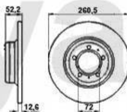
3. 610 118211 2.4 TD vorne/front
